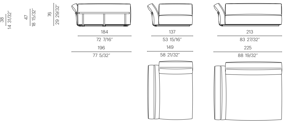
FIANCO - BRACCIOLO BASSO | END UNIT - LOW ARMREST
